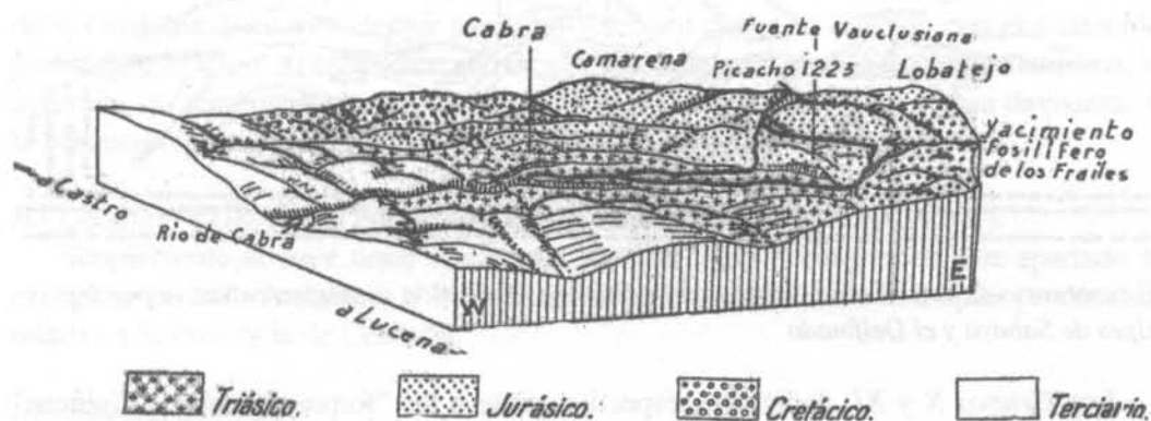
Bloque relieve de la región egabrense
