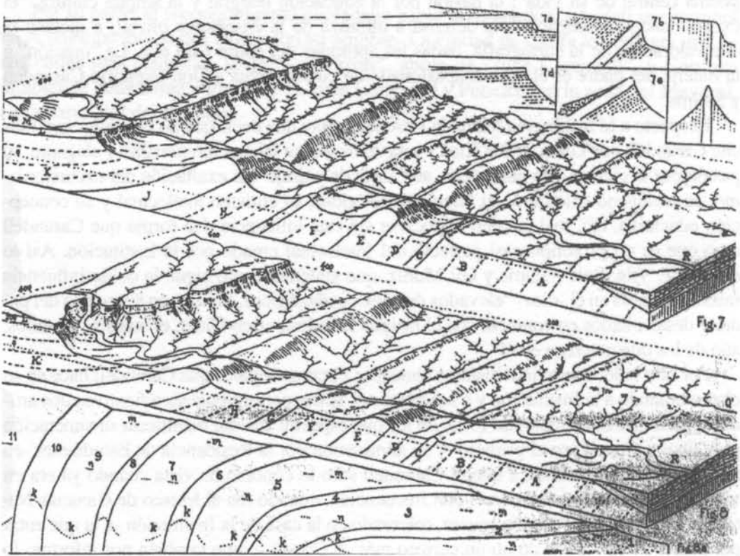
Cómo enseña Geografía el Maestro William Morris Davis. El ciclo de erosión fluvial. Figs. 7 y 8
