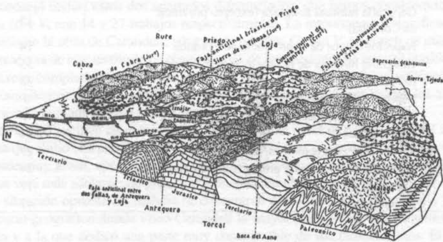
Bloque relieve de los plegamientos alpidobéticos en que está enclavado el Torcal de Antequera, con el itinerario de Cabra a Loja, Antequera y Torcal.
