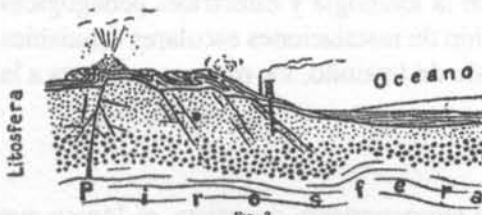
Fig. 2. Corte de la litosfera — Rocas sedimentarias plegadas o arrugadas, formando montañas. Muchas fracturas o fallas; por unas salen gases y rocas fundidas procedentes de la pirofera (volcánes); por otras, aguas termales. — En otras fracturas se han cuajado bloques volcánicos. Obsérvese cómo los ríos han depositado detritus en el fondo del océano inmediato al continente.
