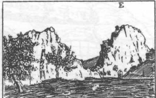
Estratos verticales, con ligero buzamiento al S W., en cuarcita silúrica. Actual cauce del Alcudía.
