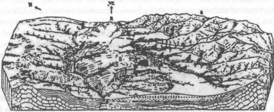
Captura del Guadalporcún por el Guadiaro (G). S. Serranía de Ronda. D. Materiales gruesos (conglomerados) depositados por el brazo del mar terciario
