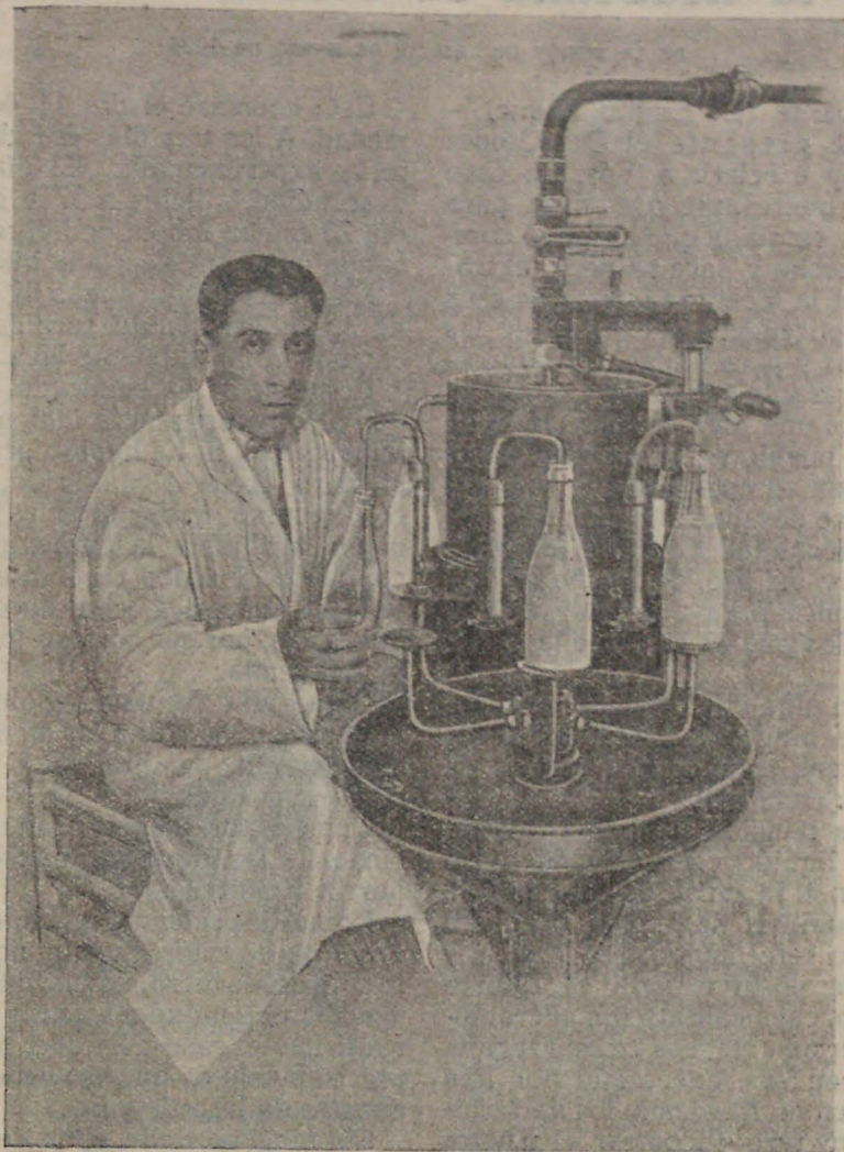
Máquina llenadora automática de botellas
