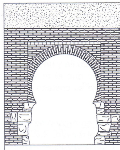
Fig.46 T.VII: Alzado Puerta Este (Nieto Medina, 2003: 259).
