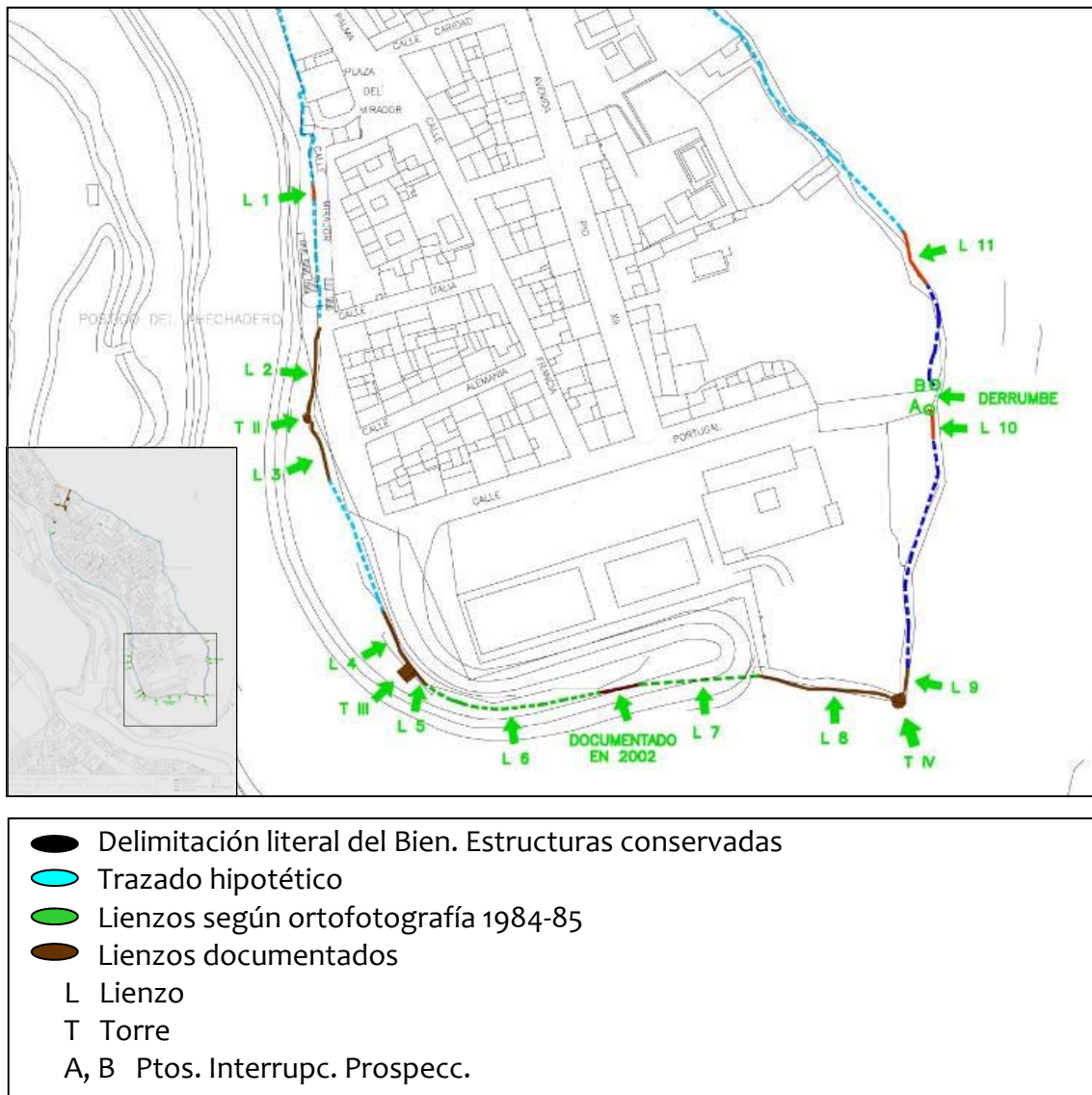
Fig.10 Pta. Gral. Rto. Amurallado. Hornachuelos. Zona S.E. (Modificado de Junta de Andalucía, 2002). E: 1/3000.
