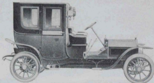
Coupé de ville 18 HP.
