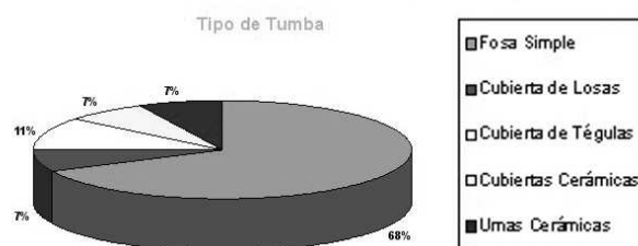
LÁMINA 5: Gráfica porcentual de los tipos de tumbas presentes en la necrópolis.
