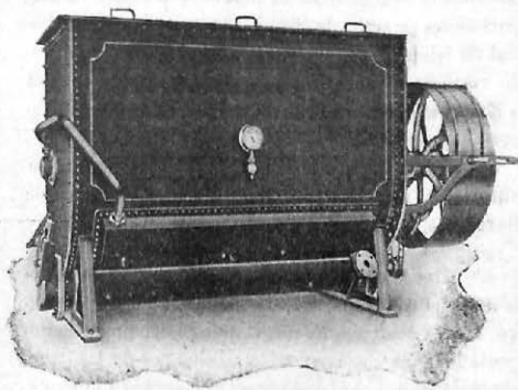
Termo-Batidor, para dar temperatura a la masa. Patente «Serraleón» de que es autor también el Sr. León Alvarez, y que constituye la base principal del nuevo molino aceitero que nos ocupa.
