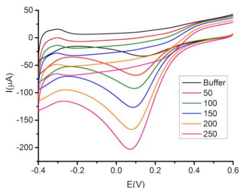
Fig. 1. Voltagramas de H_2O_2 en PBS, pH 7.0 con electrodo GC/PNR/Pt. Se añadieron volúmenes de H_2O_2 0.5M a 40 mL de tampón.
