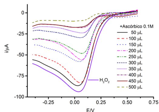
Fig. 2. Voltagramas de H_2O_2 2.98 mM en PBS, pH 7.0 con electrodo GC/PNR/Pt y volúmenes variables de ácido ascórbico añadidos a 40 mL de disolución.
