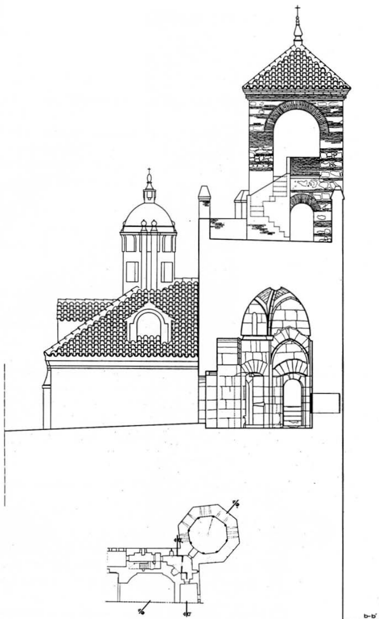
Figura 8. Plano de sección
