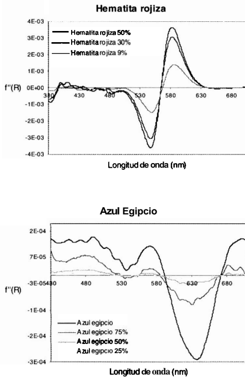
Figura 12: (Superior) Segunda derivada de la función de Kubelka-Munk para distintas concentraciones de hematita violácea. (Inferior) Segunda derivada de la función de Kubelka-Munk para distintas concentraciones de azul egipcio.
