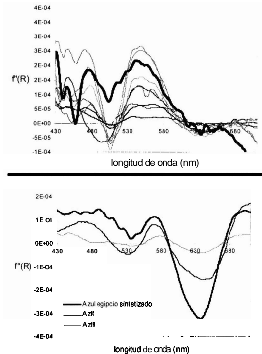
Figura 11: (Superior) Segunda derivada de la función de Kubelka-Munk de la celadonita pura (en negro) y el resto de los pigmentos verdes estudiados. (Inferior) Segunda derivada de la función de Kubelka-Munk de las muestras AzII y AzIII y del azul egipcio sintetizado en el laboratorio.
